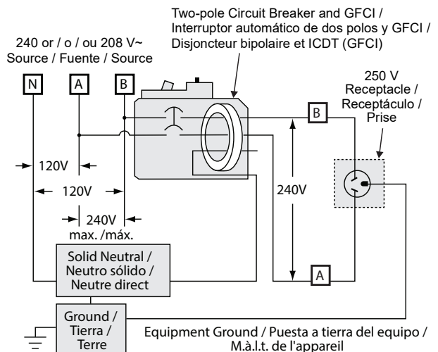
FIG. 3 : Two-wire 240 V or 208 V Circuits / Circuitos de 2 hilos de 240 V~ o 208 V~ / Circuitos à 2 fils de 240 V ou 208 V
