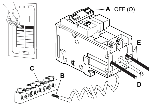
FIG. 1 : Installation / Instalación / Installation
