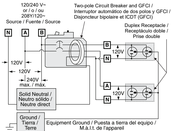
FIG. 2 : Three-wire 120/240 V or 208Y/120 V Circuits / Circuitos de 3 hilos de 120/240 V~ o 208Y/120 V~ / Circuitos à 3 fils de 120/240 V ou 208Y/120 V
