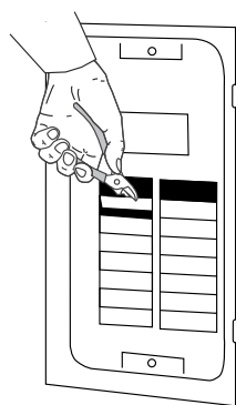
Figura 14 - Extracción de las cubiertas extraíbles
