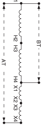
Diagrama de alambrado 4
