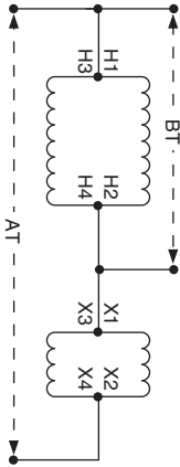
Diagrama de alambrado 1
